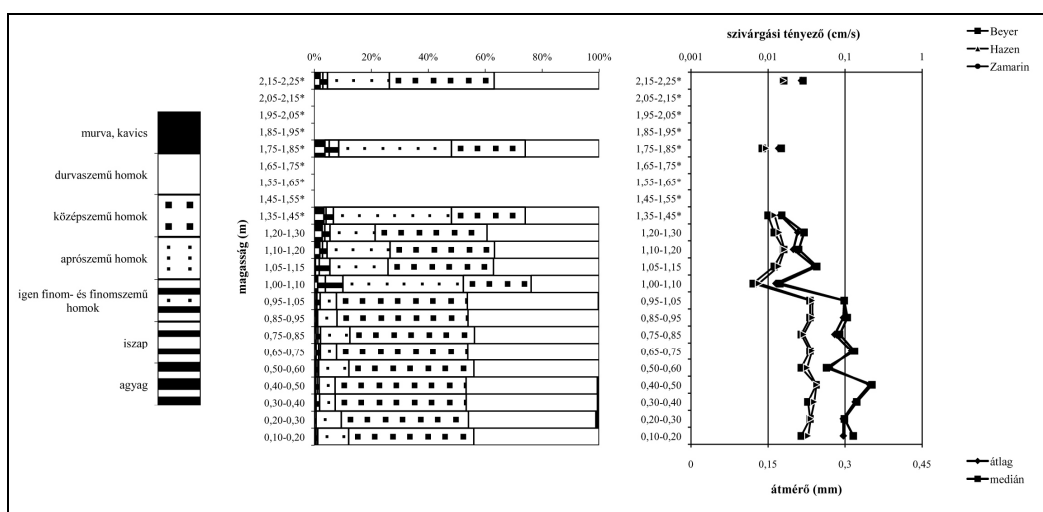
4. ábra. A szemeloszlásból számolt szivárgási tényezők, valamint az átlag és medián értékek a Nagykeréki I. és 2. szelvényből származó mintákban
