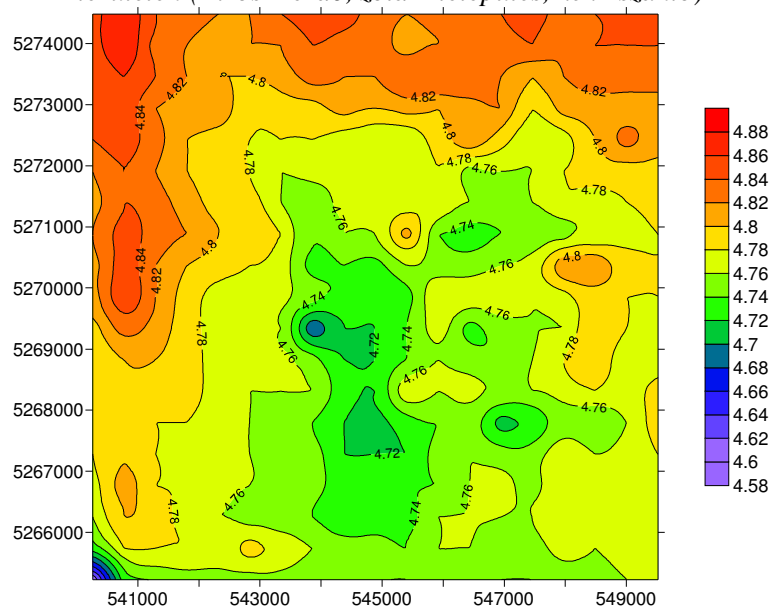
10. ábra. Szélpotenciál térkép Debrecen-Kismacs állomás környékén 50 m magasságban
