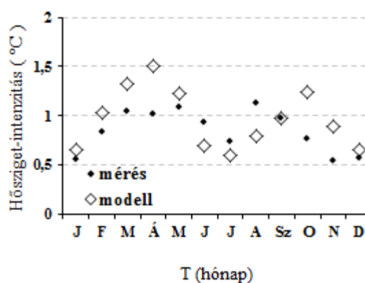
6. ábra. A modelleredményekből és a mérésekből számolt városi hősziget- intenzitás havi átlagértékei az 1999-2000. közötti időszakban Szegeden.
