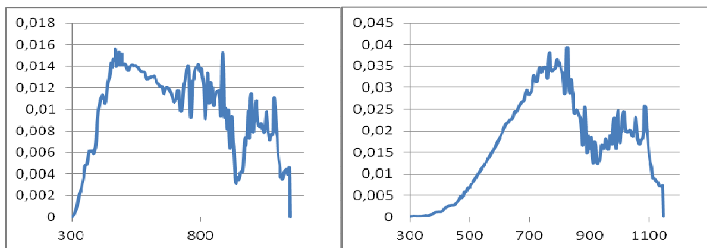
4. ábra. a) A direkt napsugárzás spektrális eloszlása egy nyári napon Debrecenben, b) Egy halogén lámpa spektruma (a vízszintes tengelyen a hullámhossz nm-ben, a függőleges tengelyen az intenzitás \text{mW}/\text{cm}^2/\text{nm} -ben)
