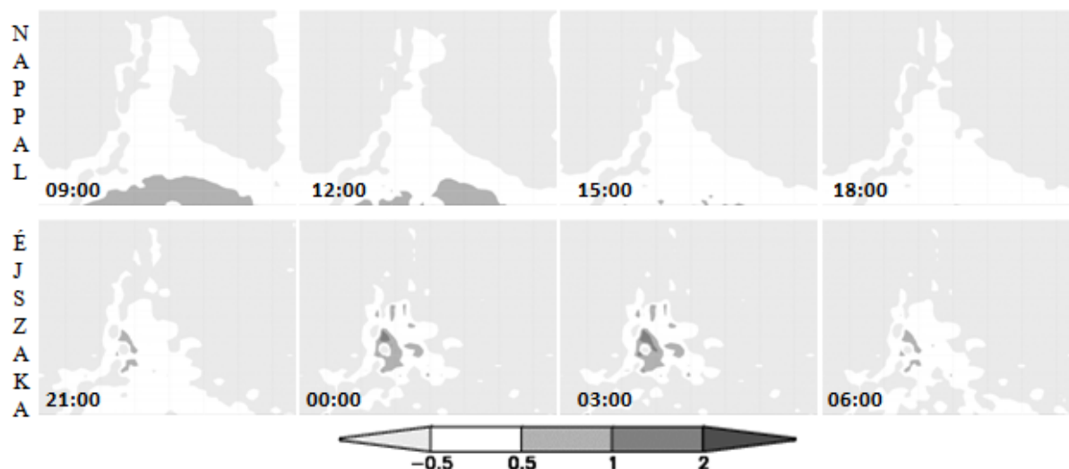
4. ábra. A júliusi átlaghőmérséklet eltérése ( ^{\circ}\text{C} ) a pestszentlőrinci rácspontban kapott értékektől a modelleredmények alapján az 1991-2000-es időszakban Budapesten és térségében a nap különböző időpontjaiban.
