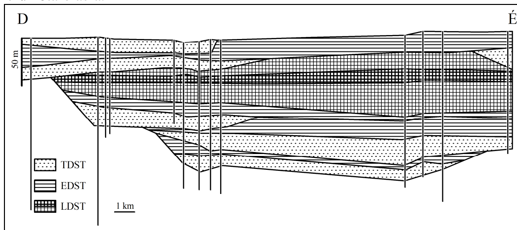
3. ábra. Szekvenciasztratigráfiai korrelációs szelvény a Hajdúháton
