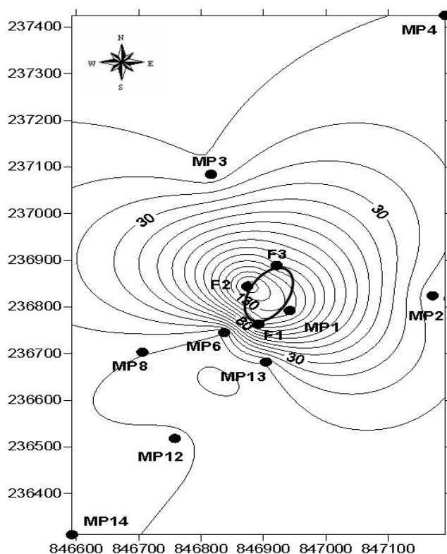
4. ábra. Az ammóniumion koncentrációjának térbeli alakulása a 12 vizsgált kút havi átlagértékei alapján 2011 novembere és 2012 szeptembere között
