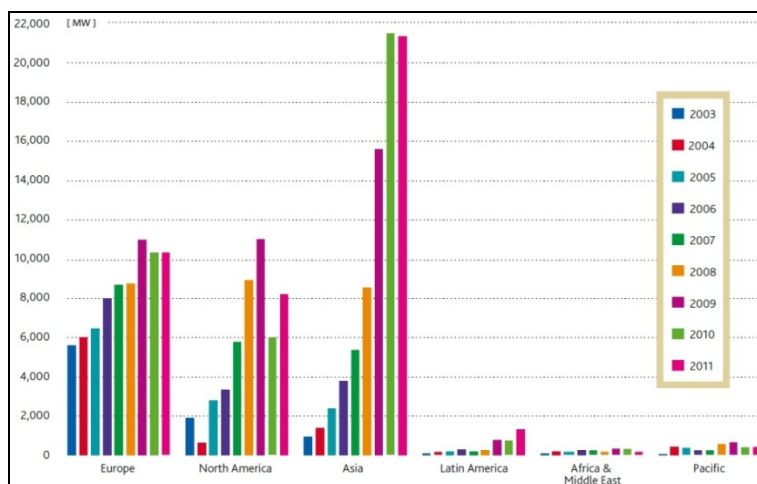
1. ábra. Évenkénti felszerelt szél erőművi kapacitás (FSZeK) 2003-2011 között
