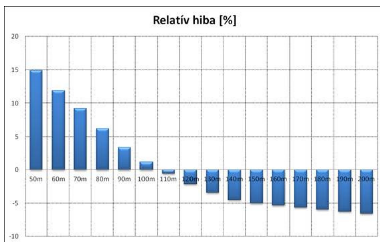
12. ábra. A mért és modellezett szélesebesség relatív hibája (%) Debrecen-Kismacs Agrometeorológiai Obszervatóriumban végzett SODAR mérések alapján (20120510-20121001)
