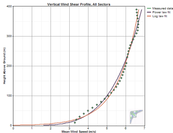
4. ábra. A szélsébség átlagos vertikális eloszlása Debrecen - Kismacs állomáson (2012.05.10-2012.10.01.)
