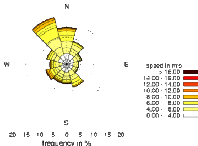
3. ábra. Szélirányonkénti szélsébség eloszlás 50 m magasságban Debrecenben (20120510-20120826)
