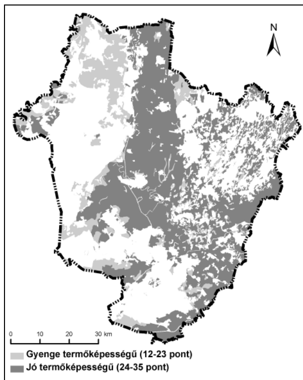
7. ábra. Cukorcirok termőhelyi alkalmasság a 2021–2050 közötti időszakra az ALADIN-Climate modell alapján
