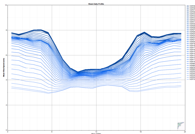
6. ábra. Az átlagos szélsébség napi menetének változása a magassággal SODAR mérések alapján Debrecenben (20120510-20121001)
