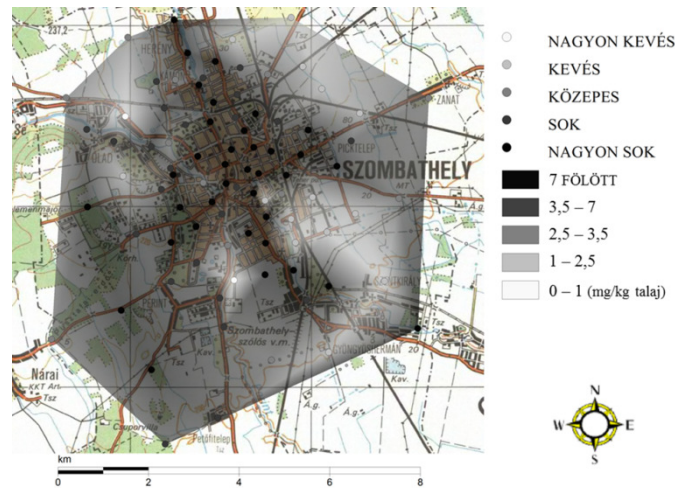
4. ábra. A cinkeredmények eloszlása 0-10 cm talajmélységben Szombathely területén.
