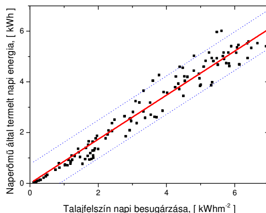
7. ábra. A pontozott vonal a 95%-os konfidencia-intervallumot mutatja, vagyis ha ismerjük a talajfelszín napi besugárzását, akkor a naperőmű által megtermelt aznapi energia 95%-os valószínűséggel a megadott intervallumba fog esni.
