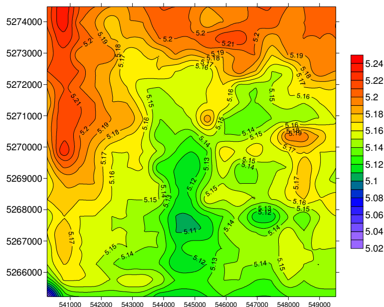
11. ábra. Szélpotenciál térkép Debrecen-Kismacs állomás környékén 100 m magasságban
