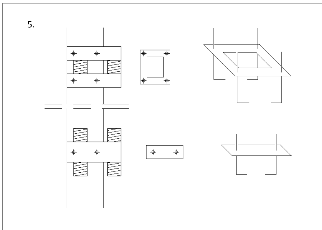
5. ábra. A tervezett épület fa tartószerkezetének és vasbeton lábazatának kapcsoló elemei
